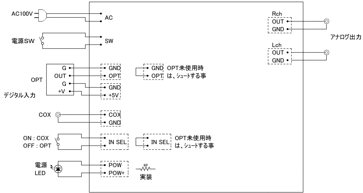
DAC Six 参考結線図
