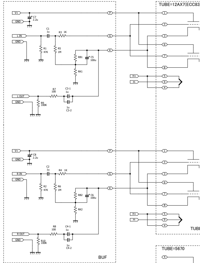
TUBE=12AX7(ECC83)
