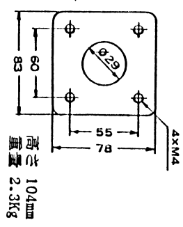
外形図
