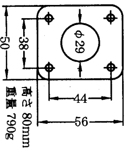
外形図
