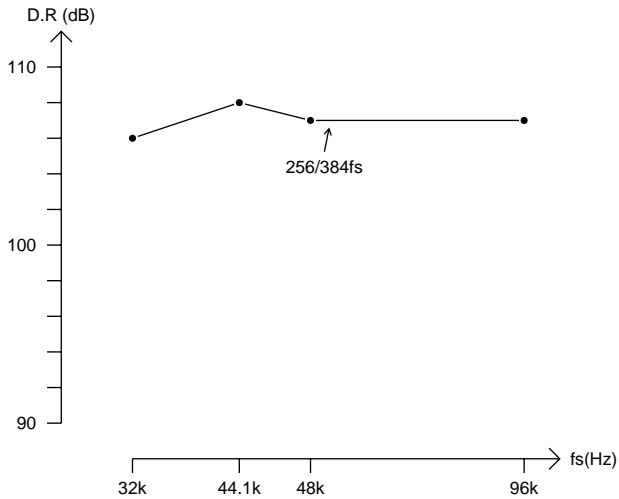
ダイナミック・レンジ対サンプリング・レート
