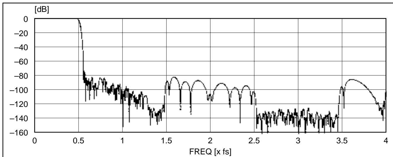
周波数特性(シャープ・ロールオフ)
