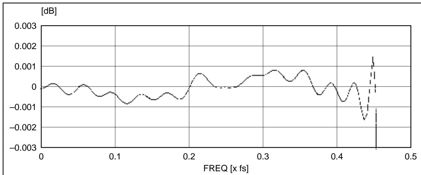
通過帯域リップル(シャープ・ロールオフ)
