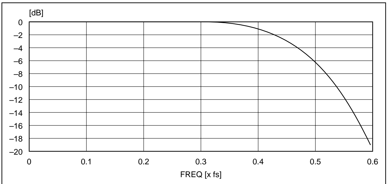
周波数特性(2)(スロー・ロールオフ)
