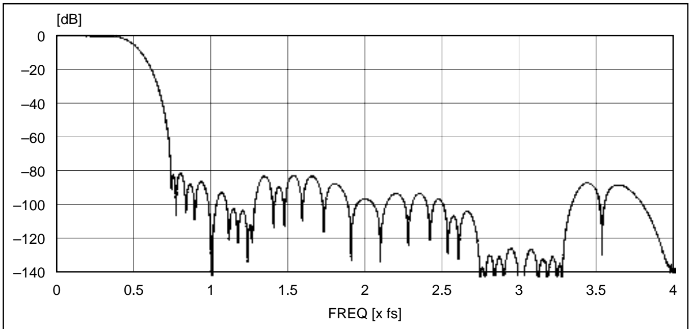
周波数特性(1)(スロー・ロールオフ)
