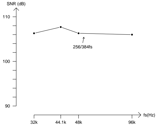
S/N比対サンプリング・レート
