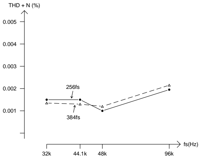
THD + N対サンプリング・レート
