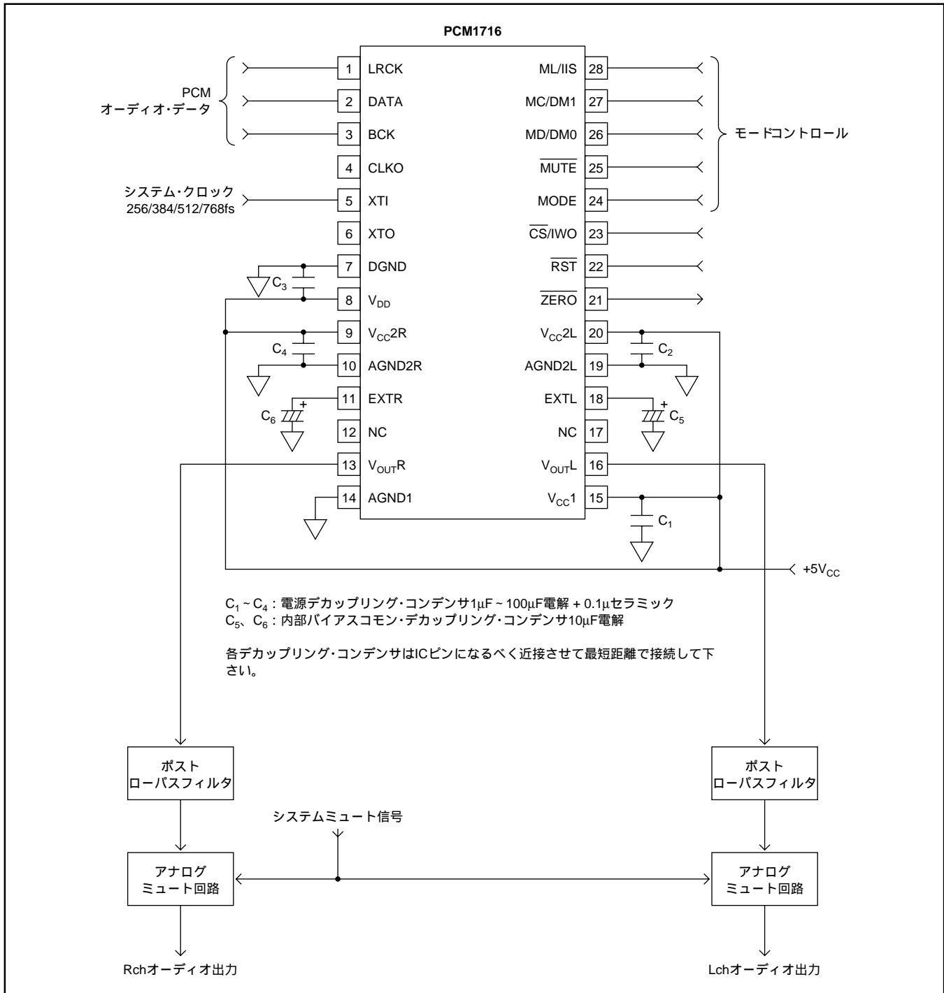
図17. PCM1716の応用接続図
