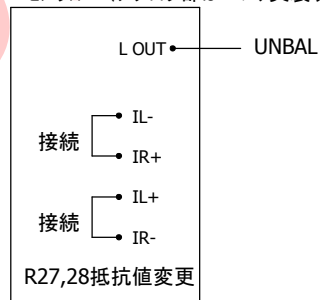
モノラル (アナログ部はLのみ実装する)
