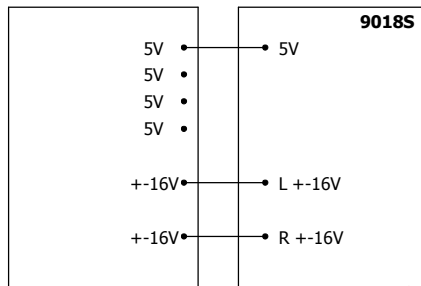
EM-PU MOS TypeBとの接続 (ステレオ設定)
