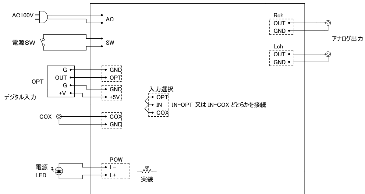
DAC Eight 参考結線図
