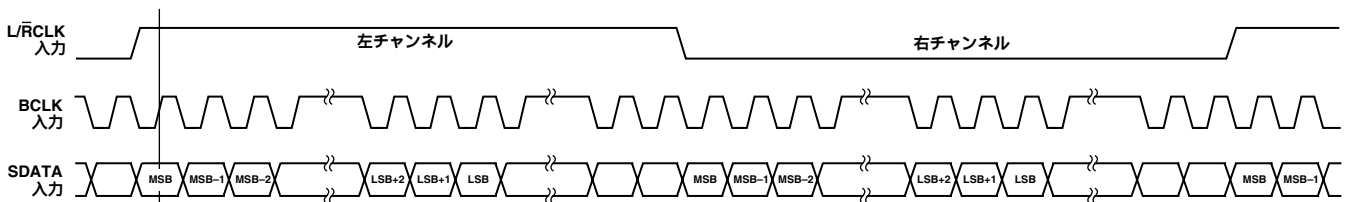
図3 左詰めモード
