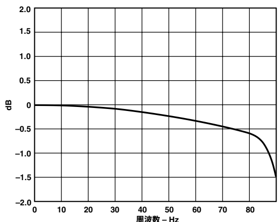
図11 2×モード、サンプル・レート192kHzでの88kHz通過帯域応答
