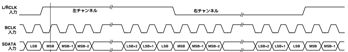
図5 32 × F s パック・モード
