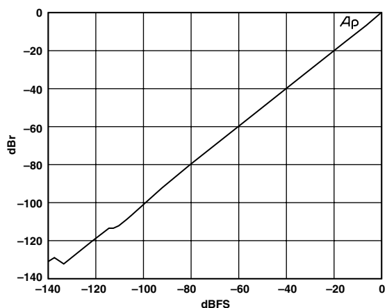
図 21 直線性 対 振幅入力 (200Hz, SR 48kS/s, 24 ビット・ワード)
