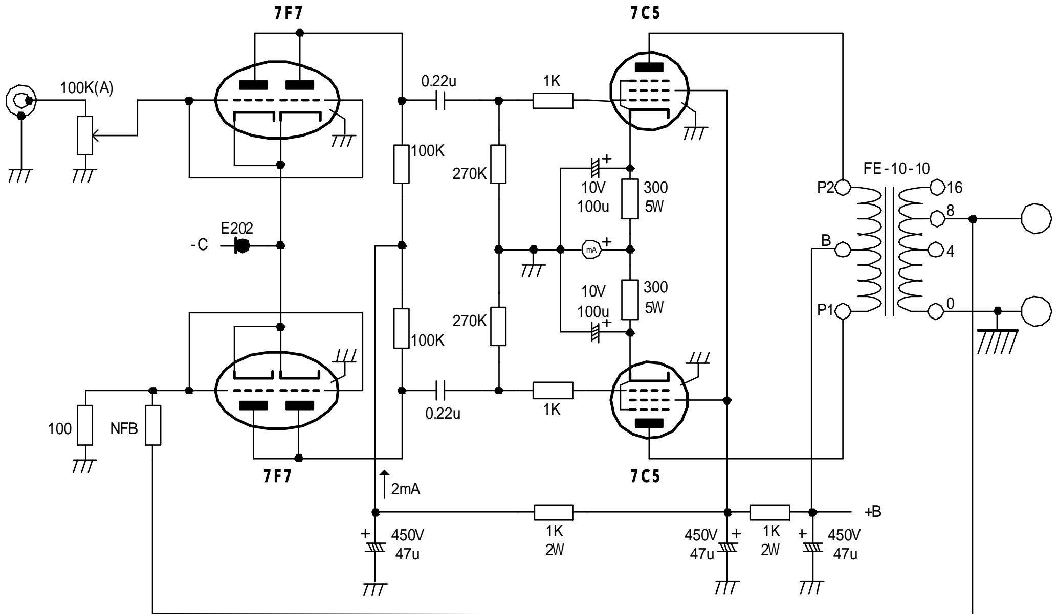
7F7 - 7C5 PP モノラルアンプ 回路図 1/2 2004/10 DESIGN BY EMISUKE
