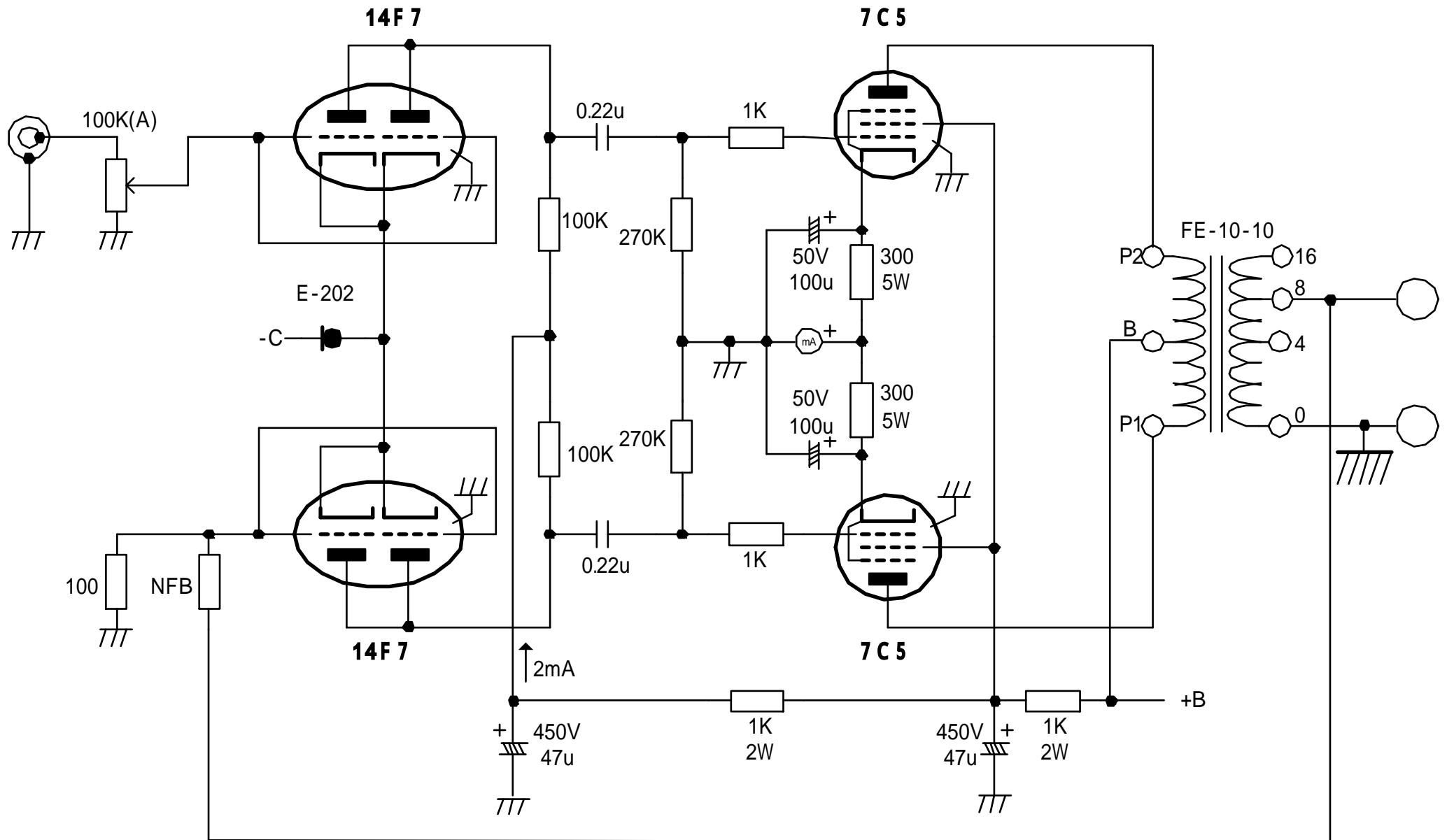
14F7 - 7C5 PP モノラルアンプ 回路図 1/2 2004/11 DESIGN BY EMISUKE
